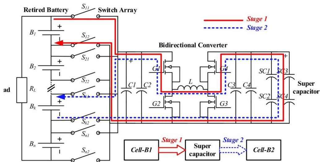
شکل ۲۳-۲ نمایی از فرآیند انتقال شارژ گروه به گروه [۶۷].
