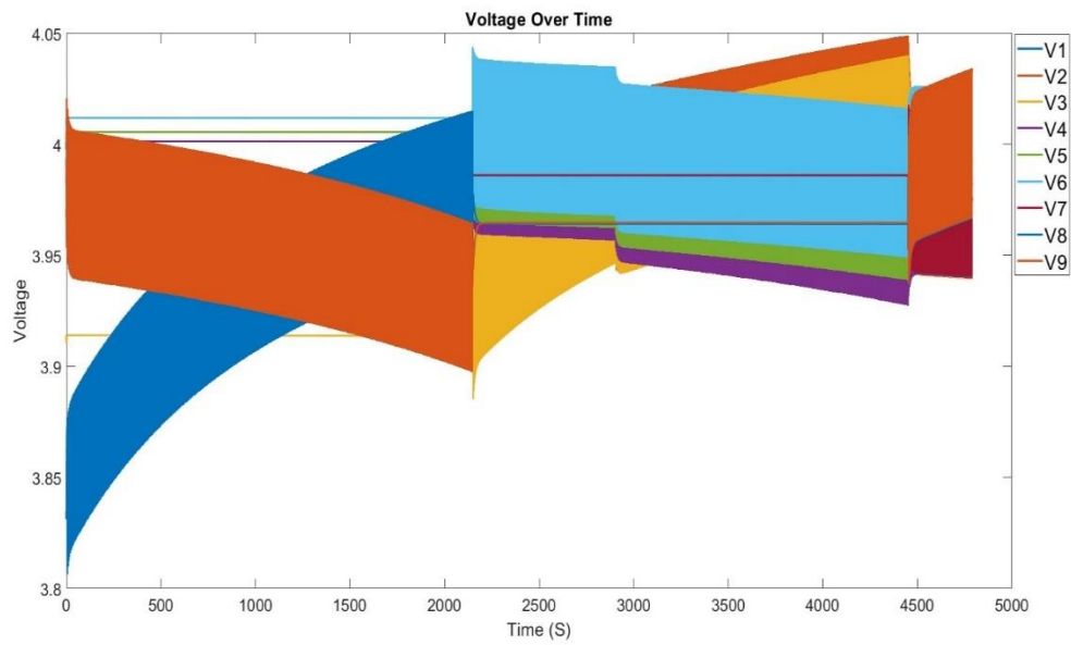
شکل ۴-۱۱ تغییرات ولتاژ سلول‌ها در فرآیند همسان‌سازی به ازای ضرایب \alpha = 0.5 و \beta = 0.5 ، \gamma = 0 .
