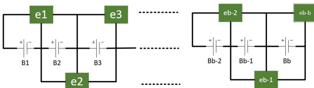
شکل ۷-۲ نمایی از توپولوژی همسان‌ساز سریالی سلول به سلول.
