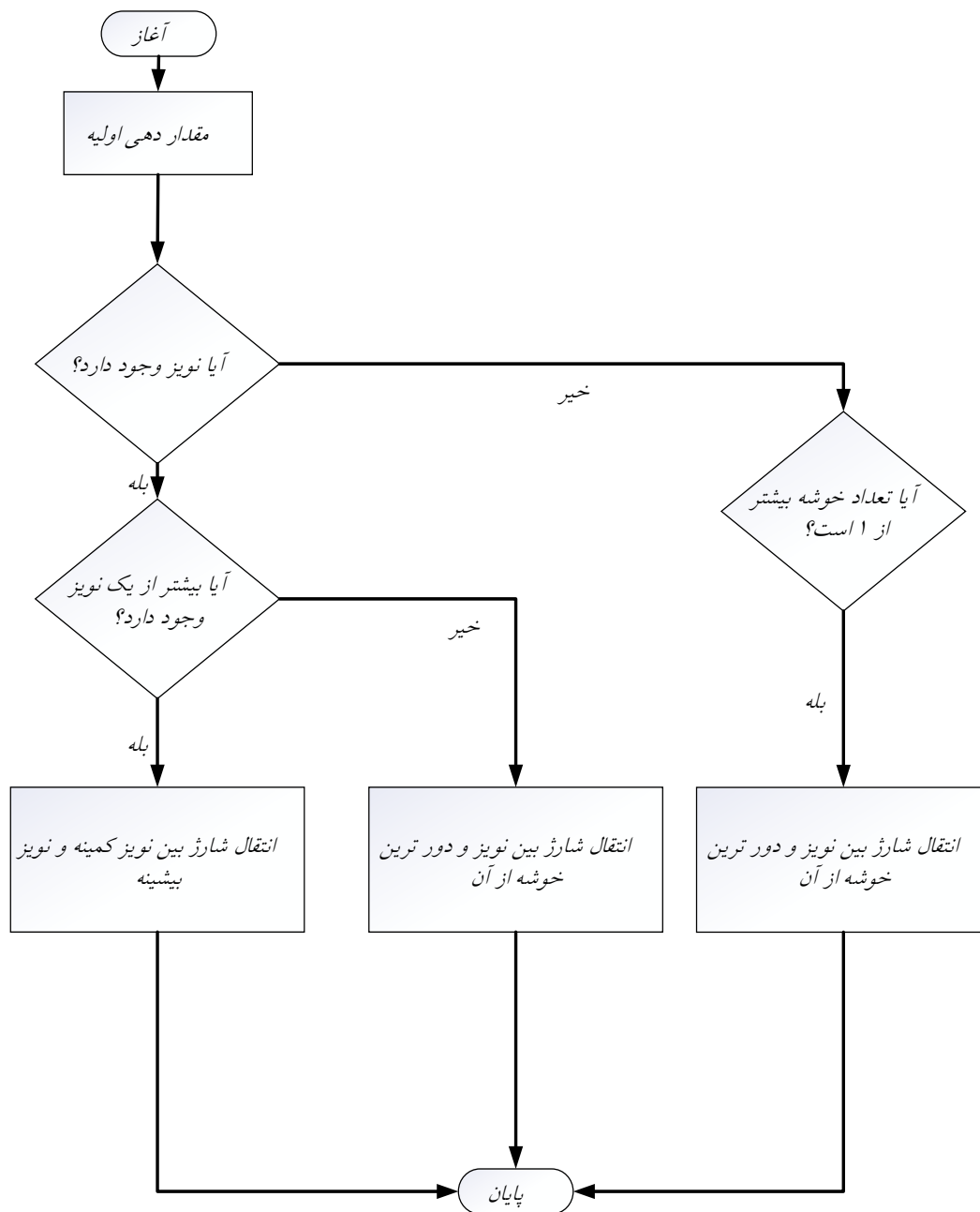
شکل ۳-۹ فلوچارت الگوریتم محاسبه‌ی همسان‌سازی سلول‌ها به صورت خوشه به خوشه، نویز به نویز و نویز به خوشه.
