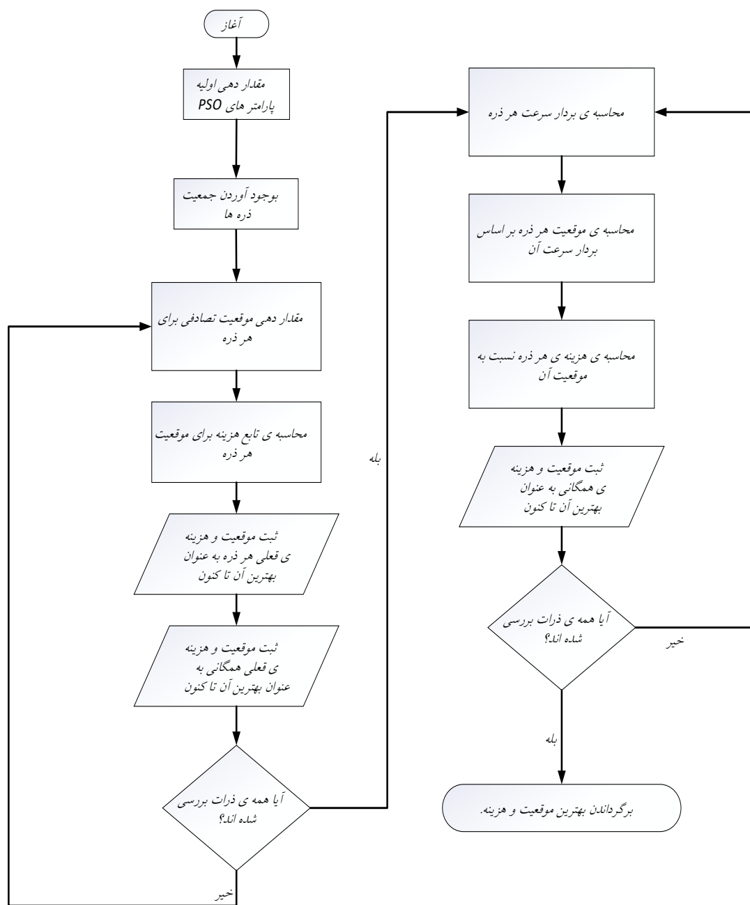
شکل ۱۱-۳ فلوجارت الگوریتم بهینه سازی ε بر اساس PSO.
