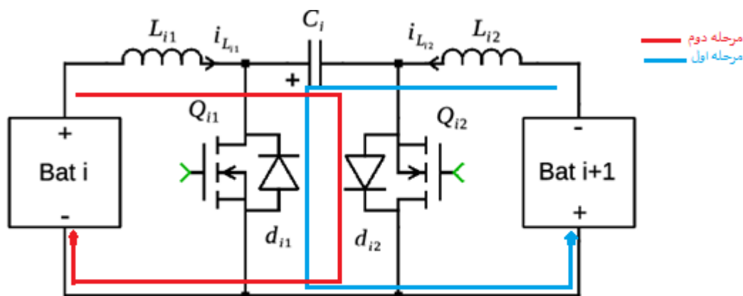
شکل ۲-۱۳ همسان‌ساز مبدل چوک [۵۴].
