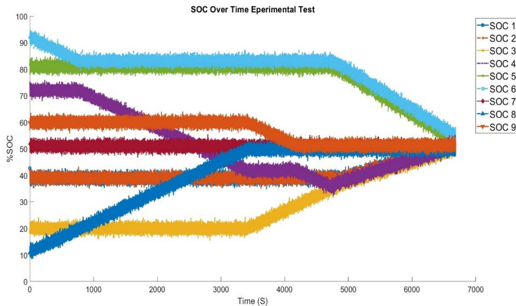
شکل ۴-۵ تغییرات وضعیت شارژ سلول‌ها در مراحل همسان‌سازی در عمل به ازای ضرایب \gamma = 0.1 ، \beta = 0.8 و \alpha = 0.1 .
