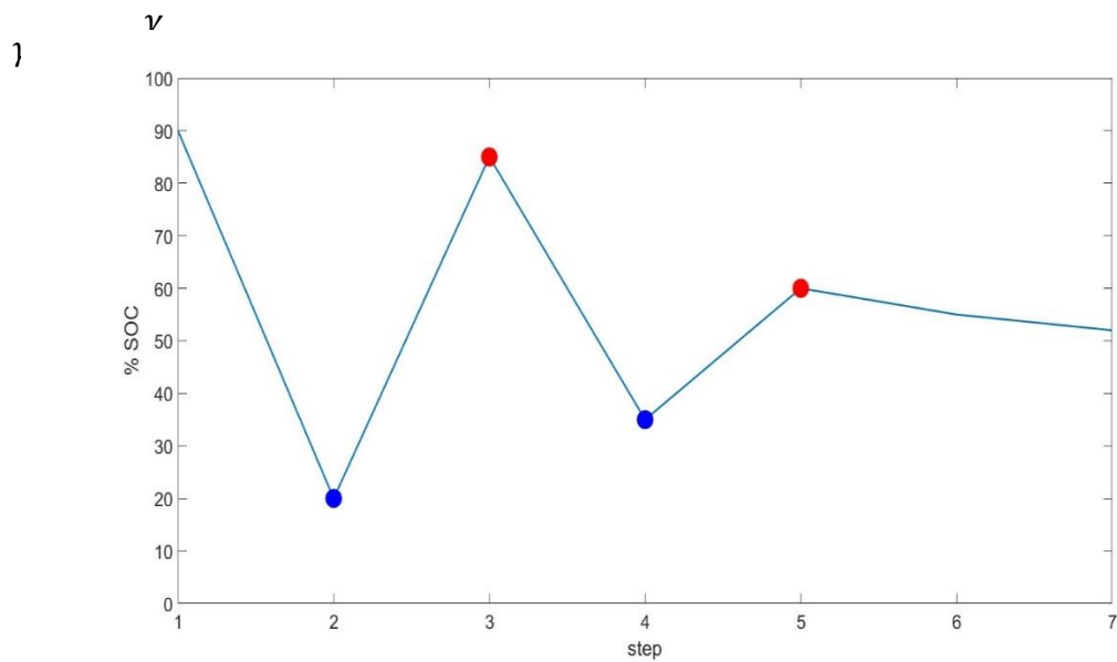
شکل ۳-۶ نمایی از تغییرات SOC یک سلول در هر مرحله از همسان سازی که در آن محل قله ها و دره ها در فرآیند روی هم رفت مشخص شده است.
