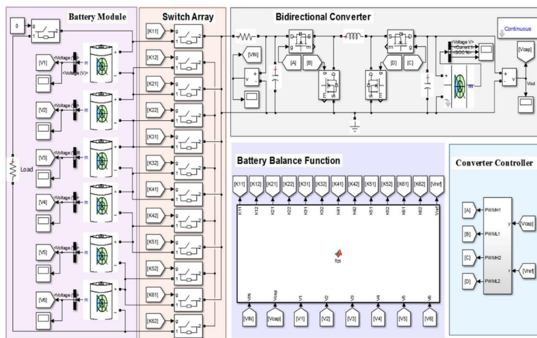
شکل ۲-۲۵ مدل شبیه‌سازی شده همسان‌ساز در متلب [۶۷].
