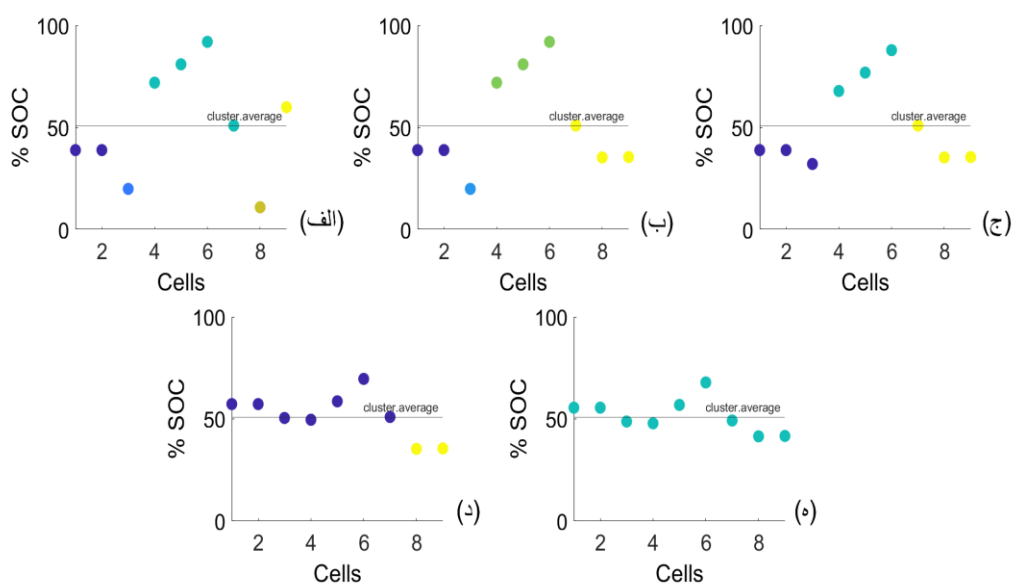
شکل ۴-۹ مراحل همسان‌سازی در پنج نوبت به ازای ضرایب \alpha = 0.5 و \beta = 0.5 ، \gamma = 0 .
