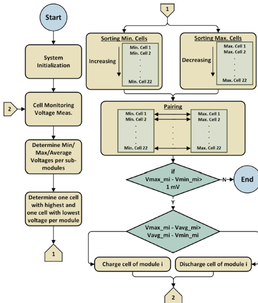
شکل ۱۷-۲ فلوجارت الگوریتم همسان سازی [۵۹].
