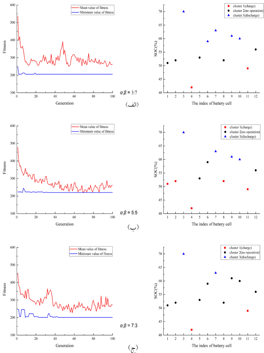
شکل ۲-۲۰ مقادیر تابع تناسب و نتایج دسته‌بندی بهینه‌شده با ضرایب متفاوت [۶۳].
