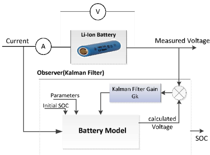
شکل ۵-۱ نمونه ساده از تخمین SOC توسط فیلتر کالمن [۲۳].
