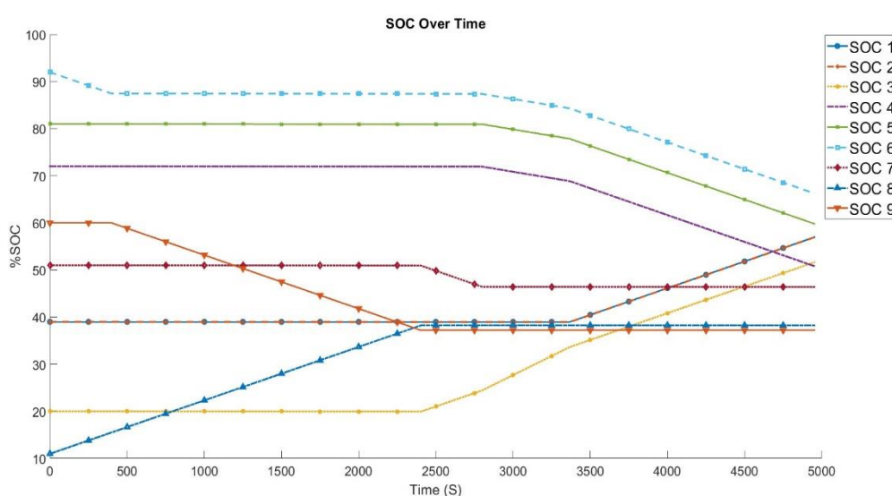
شکل ۴-۱۰ تغییرات وضعیت شارژ سلول‌ها در مراحل همسان‌سازی به ازای ضرایب \alpha = 0.5 و \beta = 0.5 ، \gamma = 0 .
