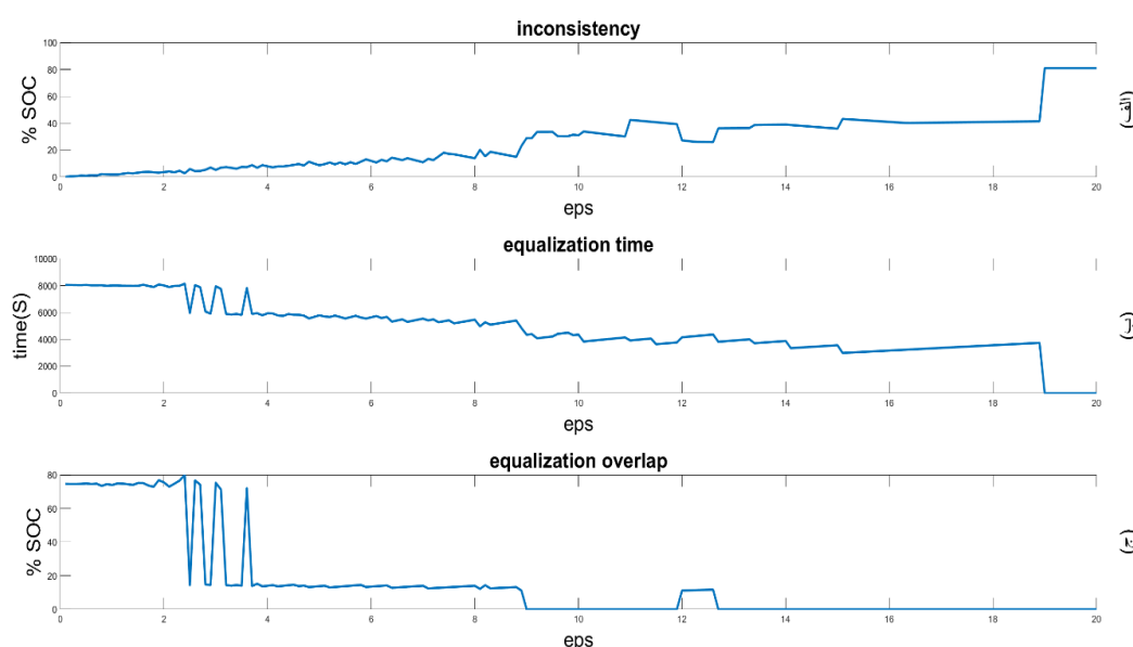
شکل ۴-۱ پارامتر \epsilon در محدوده ۰/۱ تا ۲۰ و بدون حضور PSO. عدم یکپارچگی (الف)، زمان همسان‌سازی (ب) و میزان روی‌هم‌رفت (ج).
