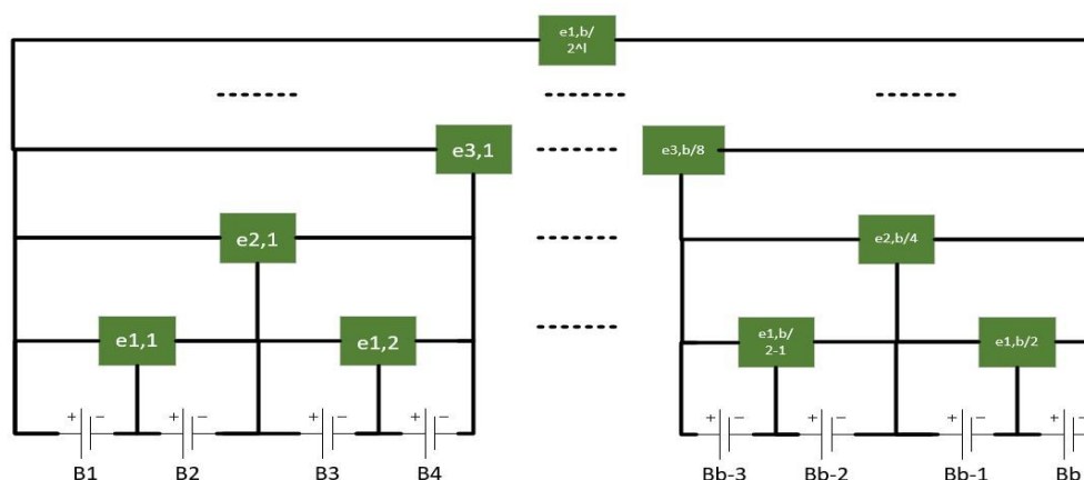
شکل ۹-۲-۱ نمای از انتقال سریالی سلول به سلول لایه‌ای.
