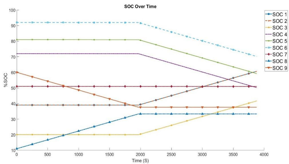
شکل ۴-۱۸ تغییرات وضعیت شارژ سلول‌ها در مراحل همسان‌سازی به ازای ضرایب \alpha = \beta = \gamma = 0.33
