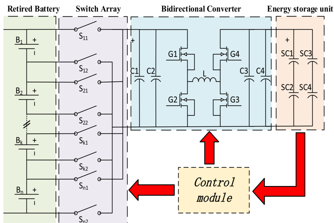
شکل ۲-۲۲ ساختار توپولوژی ارائه شده در طرح پیشنهادی [۶۷].
