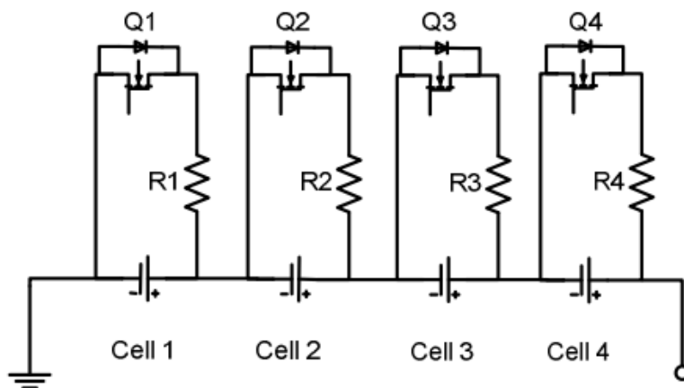
شکل ۲-۲ همسان‌سازي اتلافي با استفاده از مقاومت‌هاي شانت [۳۴].
