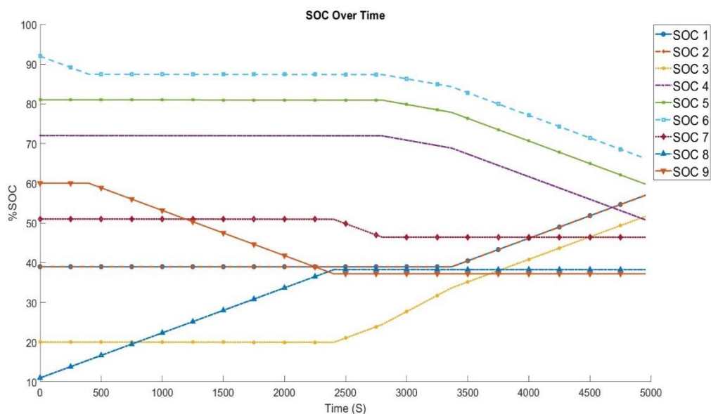
شکل ۴-۱۴ تغییرات وضعیت شارژ سلول‌ها در مراحل همسان‌سازی به ازای ضرایب \alpha = 0 و \beta = 0.5 ، \gamma = 0.5 .
