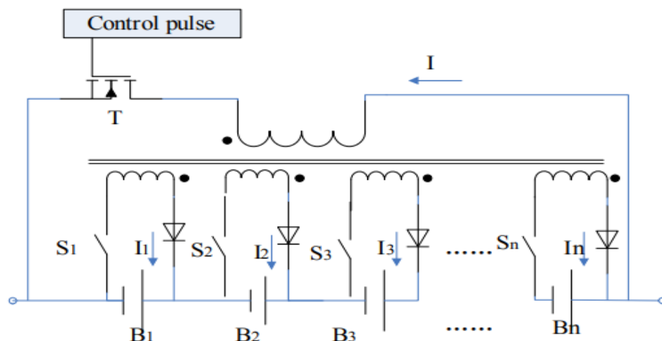
شکل ۲-۱۴ ساختار یک همسان‌ساز بر مبنای ترانسفورماتور چندسیم‌پیچ [۵۵].
