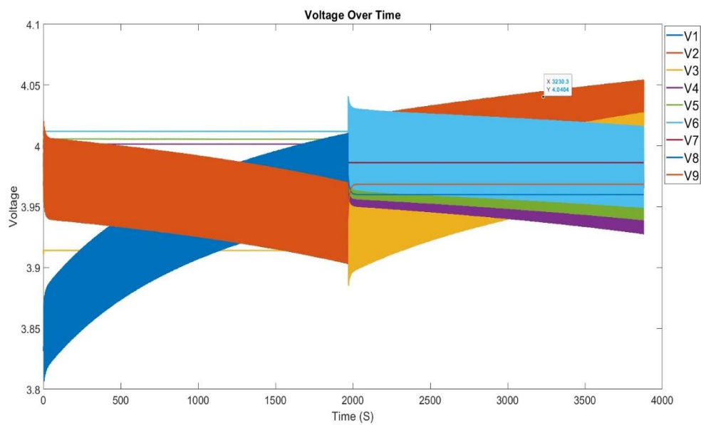
شکل ۴-۱۹ تغییرات ولتاژ سلول‌ها در فرآیند همسان‌سازی به ازای ضرایب \alpha = 0 و \beta = 0.5 ، \gamma = 0.5 .
