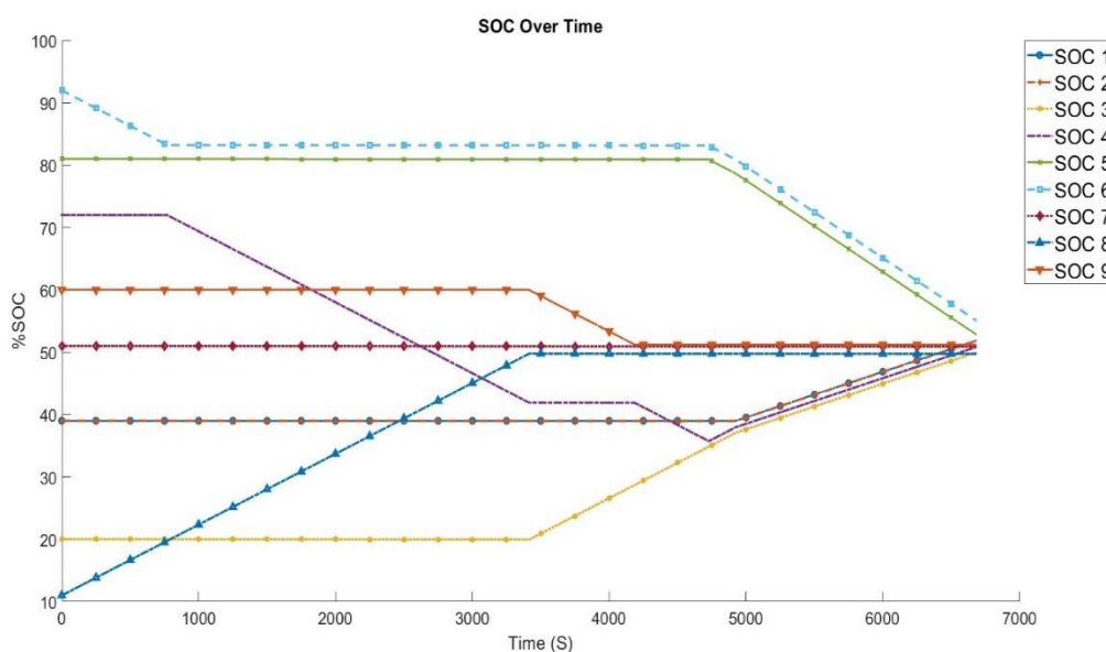
شکل ۴-۴ تغییرات وضعیت شارژ سلول‌ها در مراحل همسان‌سازی به ازای ضرایب \alpha = 0.1 و \beta = 0.8 ، \gamma = 0.1
