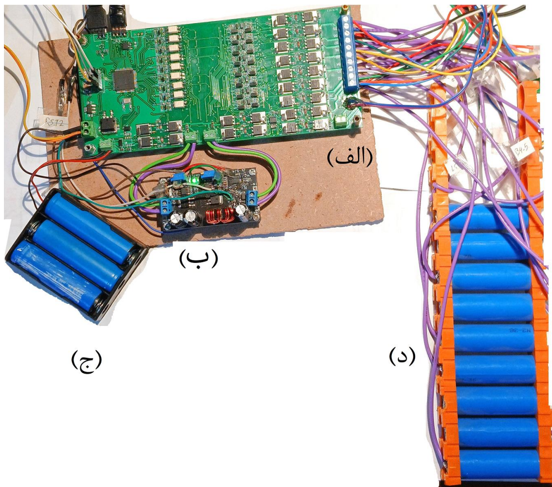
شکل ۳-۱۶ پیاده‌سازی عملی همسان‌ساز پیشنهادی (الف) برد سخت‌افزاری، (ب) مبدل جریان مستقیم، (ج) تانک انرژی و (د) پک باتری.
