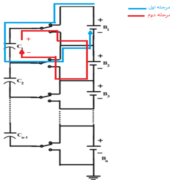
شکل ۲-۱۵ ساختار مدار همسان سازی بر مبنای سوئیچ خازنی [۵۳].
