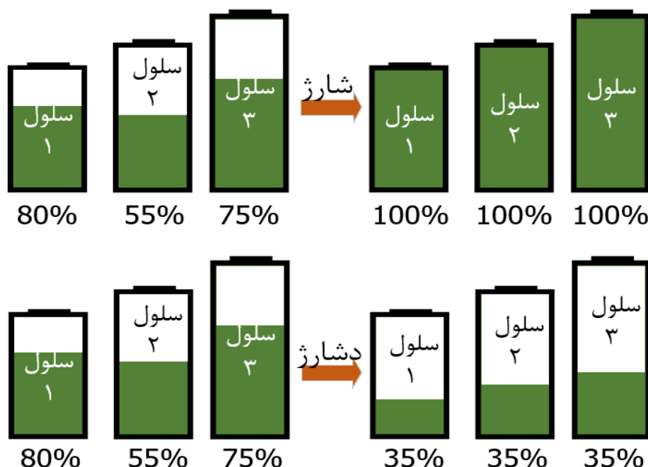
شکل ۲-۴ همسان‌سازی مبتنی بر SOC پک باتری در فرآیند شارژ و دشارژ.
