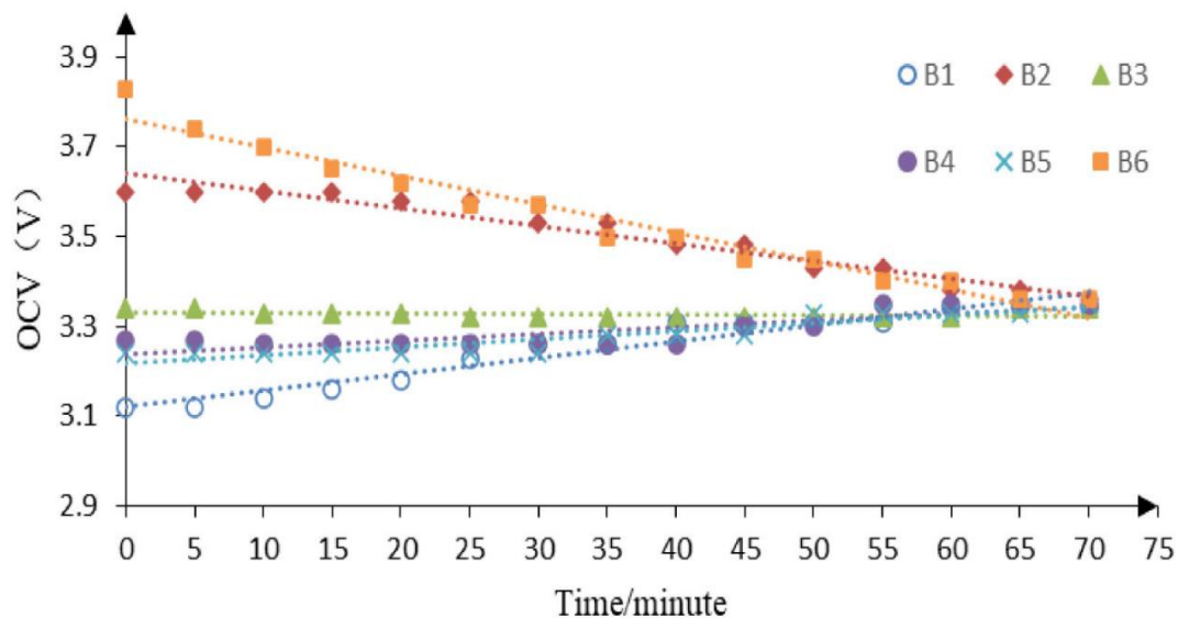
شکل ۳-۱۸ نمودار خروجی ولتاژ باتری‌ها در فرآیند همسان‌سازی با روش DBSCAN [۶۷].
