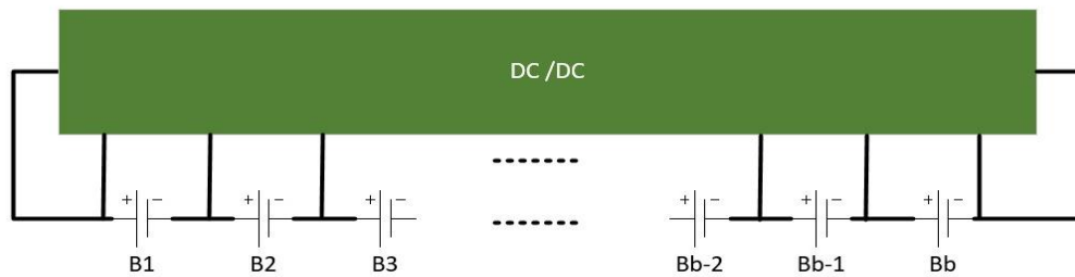
شکل ۱۰-۲ نمایی از انتقال سریالی سلول به پک باتری.
