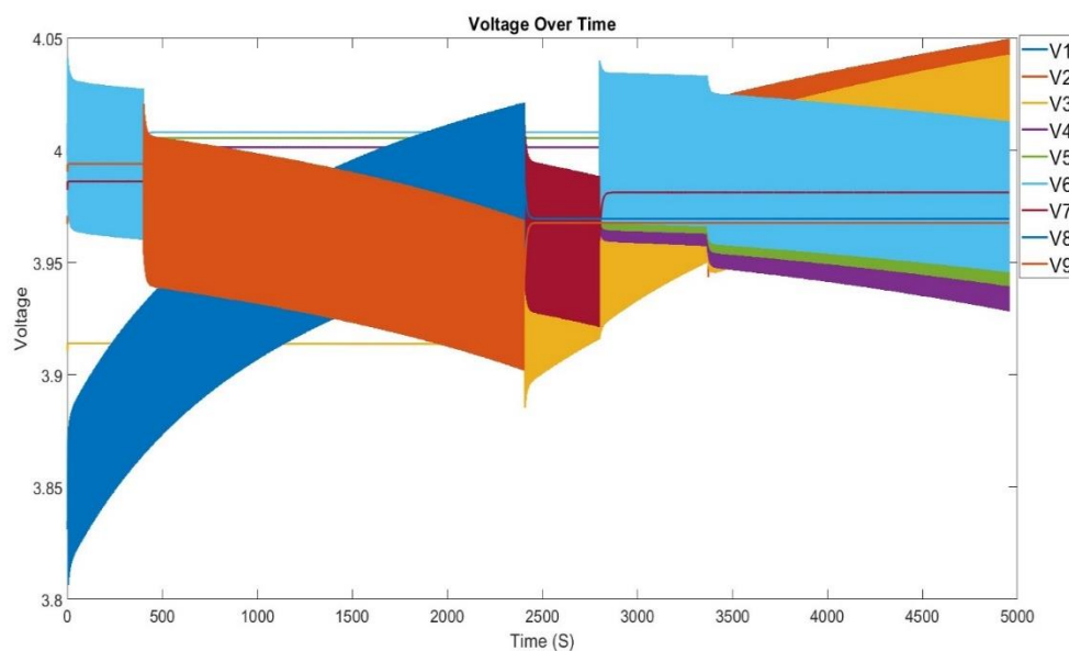
شکل ۱۵-۴ تغییرات ولتاژ سلول‌ها در فرآیند همسان‌سازی به ازای ضرایب \alpha = 0 و \beta = 0.5 ، \gamma = 0.5 .
